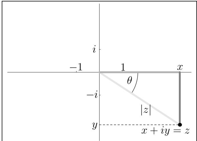
Fig. 2: x > 0, y < 0, -\pi/2 < \theta < 0
