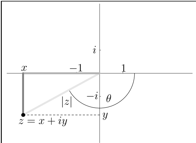
Fig. 1: x < 0, y < 0, -\pi < \theta < -\pi/2
